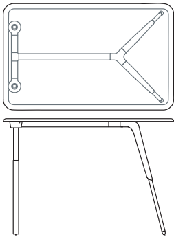
Backbone for rectangular meeting table 1BE0411: L 63 D 39½ H 43¼ 1BE0416: L 71 D 39½ H 43¼ 1BE0421: L 78¾ D 39½ H 43¼
