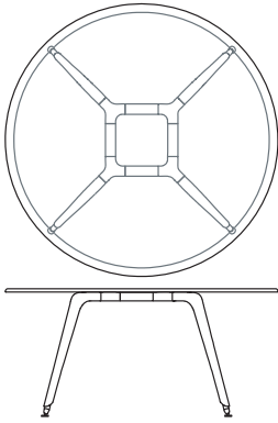
Round meeting table 1BE0431: L 55 D 55 H 29½ 1BE0435: L 63 D 63 H 29½
